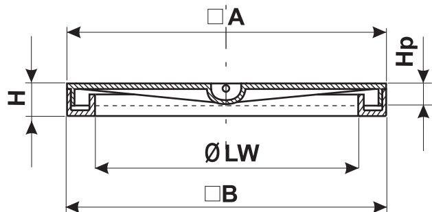
Presjek A-A:
